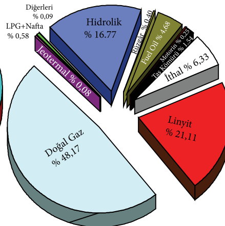
GRAFİK 4: Üretimin Kaynaklara Göre Değişimi (2008)
